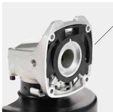
添加散热板
